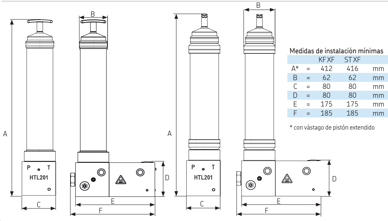
Medidas de instalación mínimas depósitos KF XF y ST XF Fig. 6
